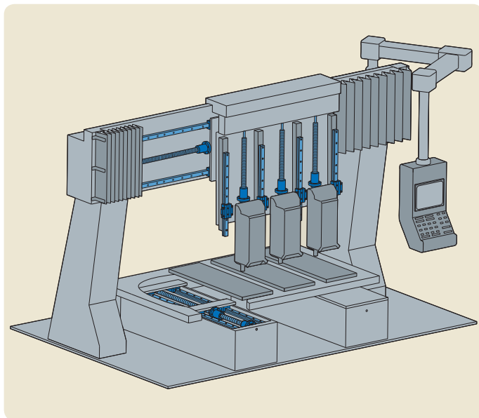
Zastosowane komponenty a) Szlifowane śruby kulkowe
