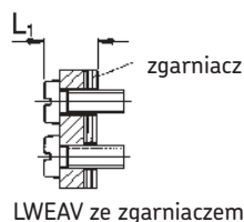
LWEAV ze zgarniaczem
