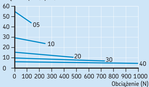
Prędkość w funkcji Obciążenia (siły)
