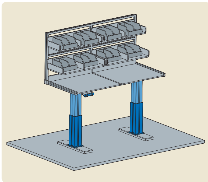
Zastosowane komponenty a) Kolumny teleskopowe b) Wyłącznik pulpitowy
