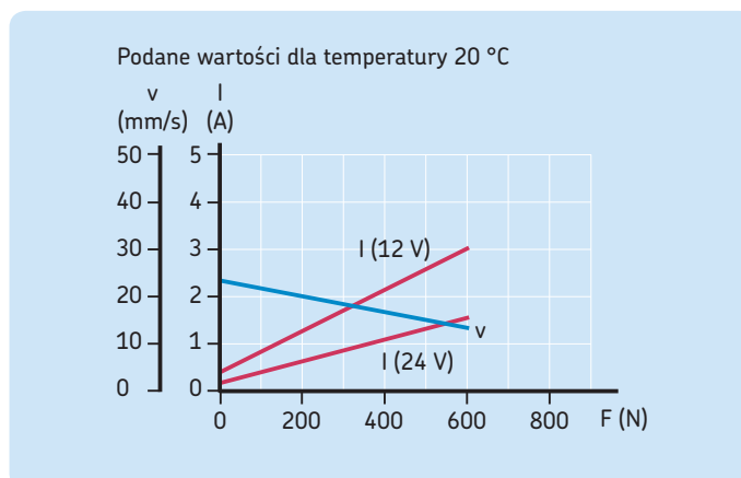
Wykres osiągow eksploatacyjnych
