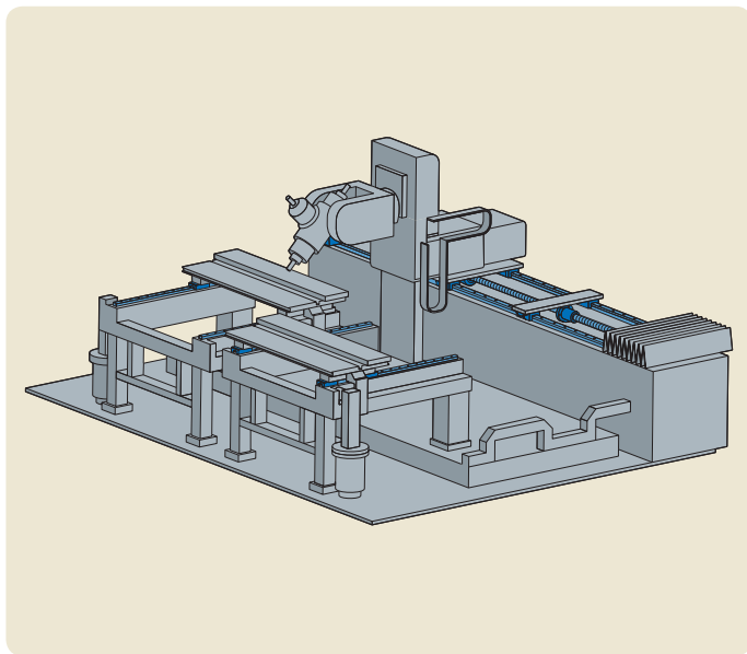
Zastosowane komponenty a) Profilowane prowadnice szynowe b) Precyzyjne śruby kulkowe
