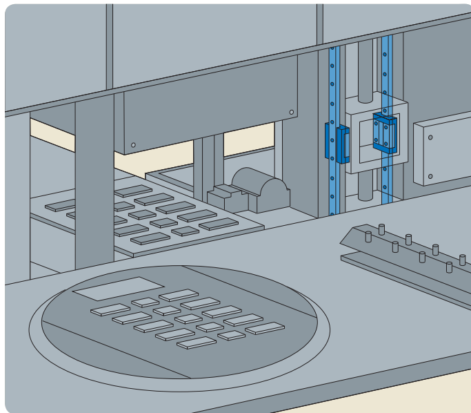
Zastosowane komponenty a) Profilowane prowadnice szynowe
