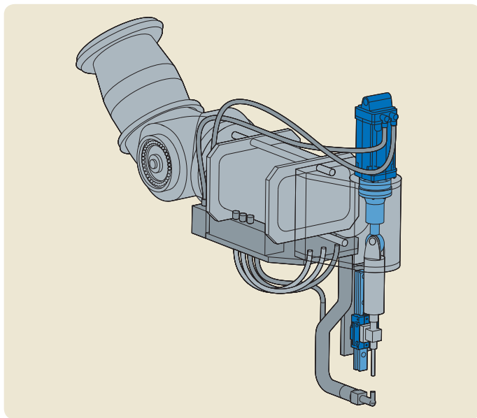
Zastosowane komponenty a) Kompaktowy cylinder elektromechaniczny
