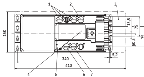
Widok bez pokrywy zabezpieczającej
